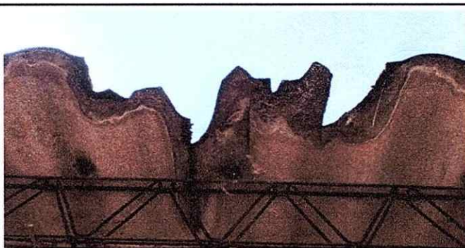
Foto 5: se Observa el deterioro de las laminas y estructuras metalicas del modulo 2
