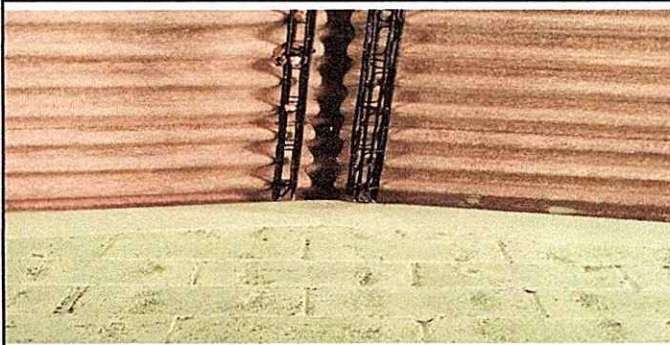
Foto 3: Se observa el capote de las laminas deteriorado modulo 1
